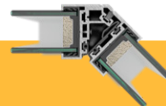
135° DETALLE UNIÓN
