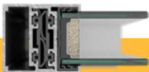
DETALLE UNIÓN PERFIL LATERAL
